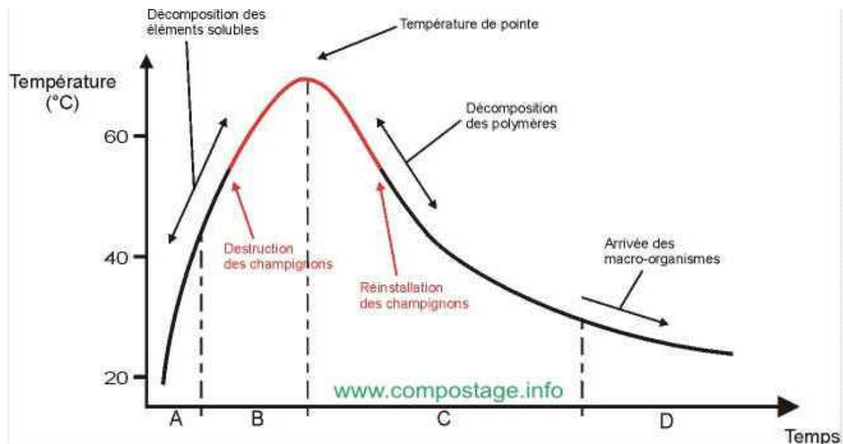
Figure n°2 : Evolution des températures au cours du compostage d'effluents de ferme (Source : www.compostage.info ).
